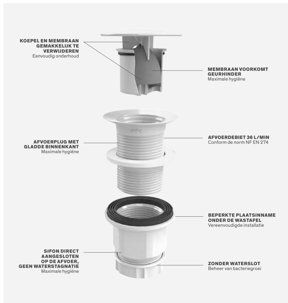
Doorsnede 621W: waterloze afvoerplug Ref. DELABIE : Coupe3D_621W
