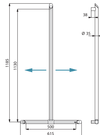
Plaatsing van de verticale stang is regelbaar
