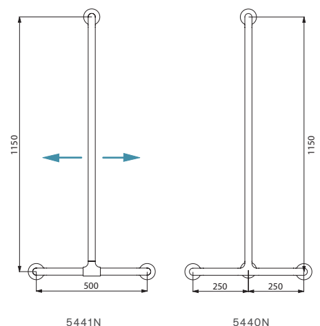
Plaatsing van de verticale stang is regelbaar (ref. 5441N)
